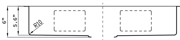
Section A-A
